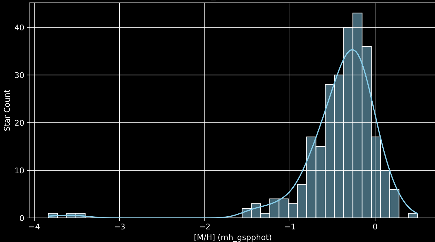
GALAH DR4 Field: [9094] [M/H] (mh_gspphot) (n= 270)
