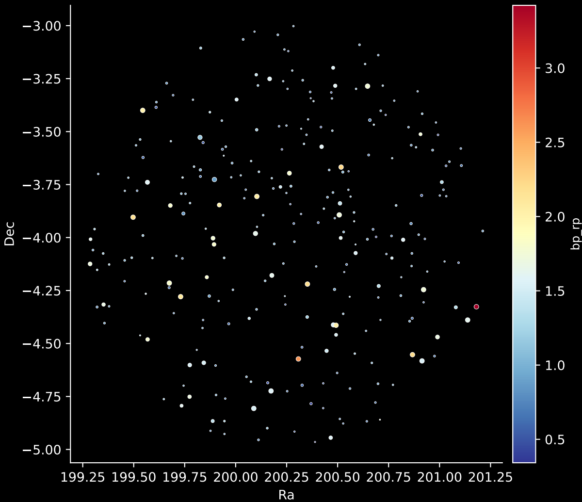
GALAH DR4 Field: [9094] Stars: 270
