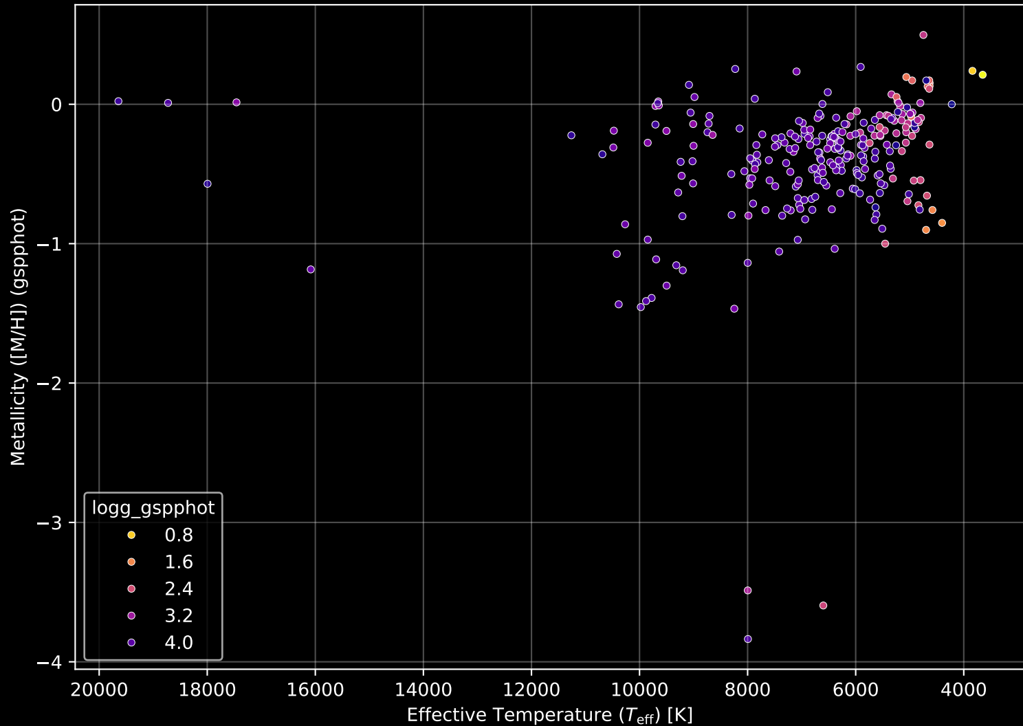
GALAH DR4 Field: [9094] Stellar Population Parameters (n= 270)
