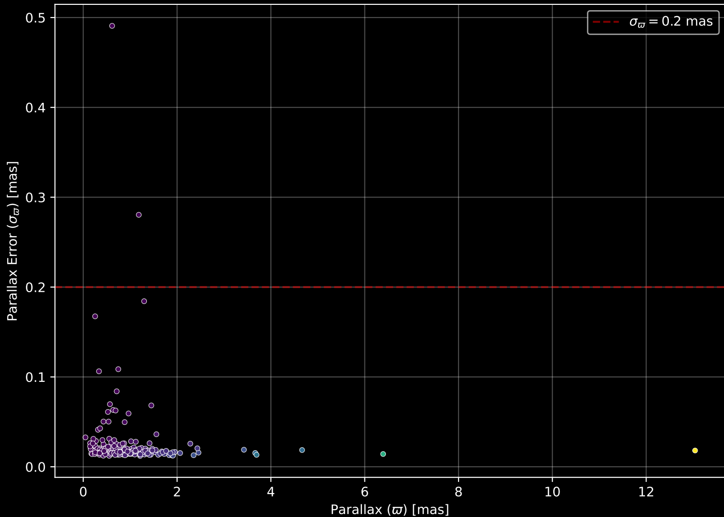
GALAH DR4 Field: [9094] Parallax Quality (n= 270)
